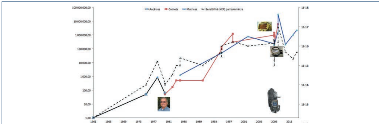
Figure 2. Diagramme schématique des lignées techniques des bolomètres, les premiers modernes qualifiés d'ancêtres, puis la lignée à cornets, débutant quelques années après l'invention des cônes de R. Winston en 1970, et enfin celle des bolomètres organisés en matrices. Le niveau de performance (à gauche en ordonnée) est le nombre de bolomètres (dans l'instrument) multiplié par l'efficacité (ouverture efficiency) divisé par la sensibilité (Noise Equivalent Power, NEP) des bolomètres individuels. Ce niveau de performance permet de comparer des caméras de bolomètres. Les courbes de performances des lignées "cornets" et "matrices" se rejoignent en 2009 avec les instruments SPIRE et PACS du satellite Herschel. À titre comparatif, la courbe hachurée représente l'évolution du NEP (à droite en ordonnée). Les photos de R. Winston et des instruments sont placées sur la chronologie.
